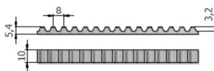
CORREA TIPO ISO 13050 R8M
