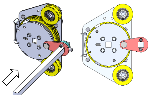
TRASMISSION EXTERIEURE À L'AXE
