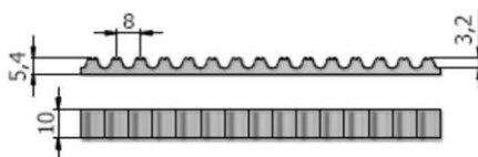
CINGHIA DENTATA TIPO ISO 13050 R8M
