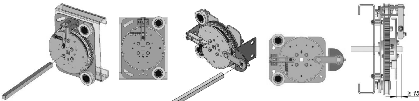
TRASMISSIONE SULL'ALBERO
